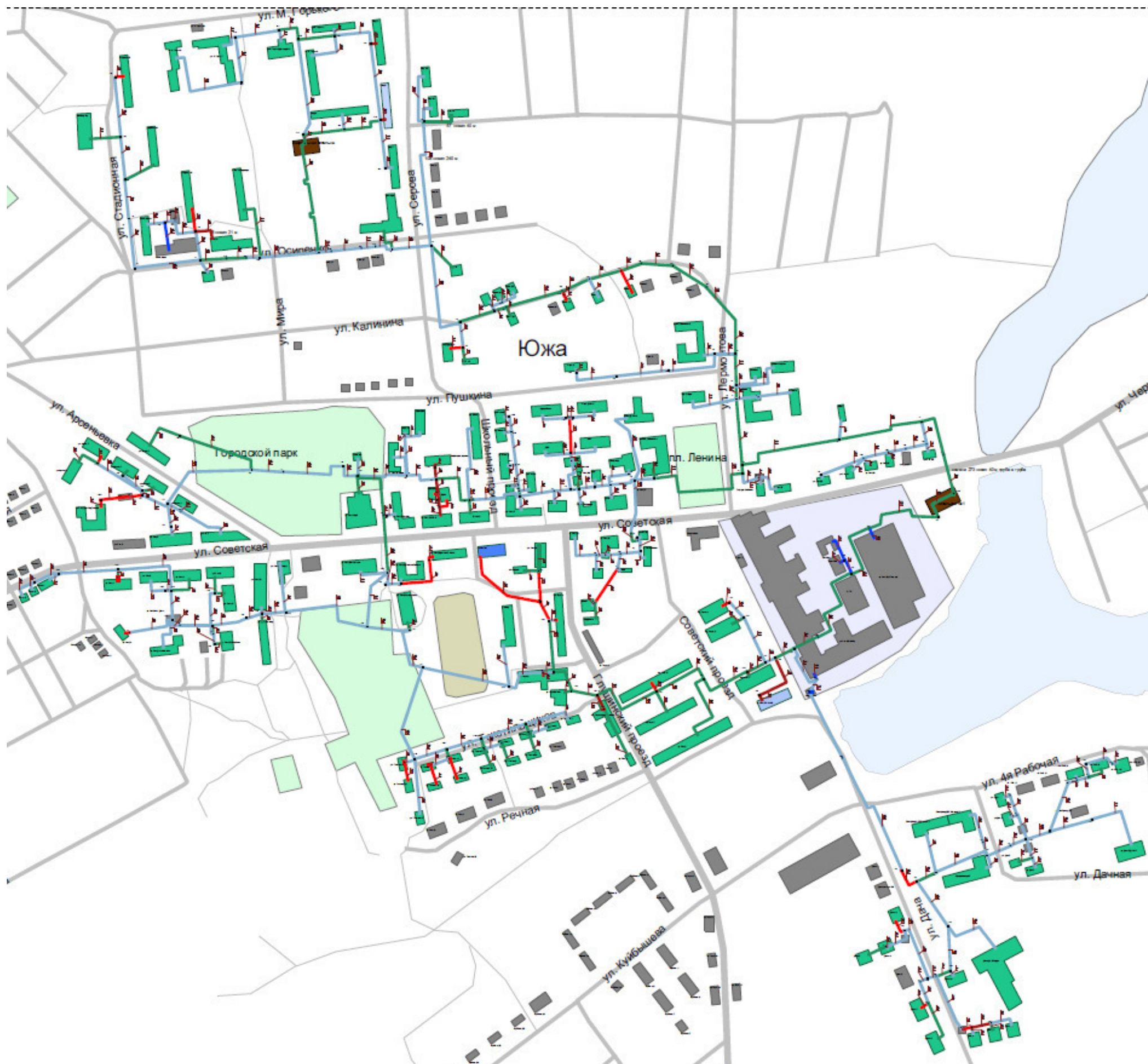
Рис. 5.1.2. Наладка теплогидравлического режима по средствам установки дроссельных сужающих устройств при температурном режиме 95/70 и замене участка тепловой сети.
